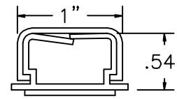
P/N: FWH-10060 BASE
